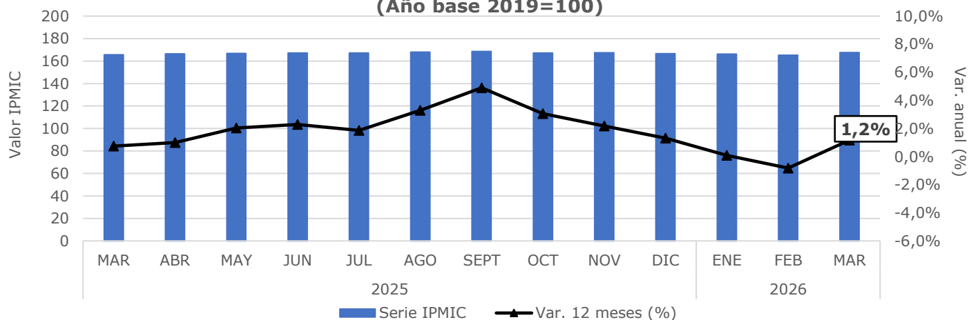
Índice de Precios de Materiales e Insumos de Construcción (IPMIC), Valor índice y variación porcentual respecto igual mes año anterior, período marzo 2025-marzo 2026 (Año base 2019=100)
