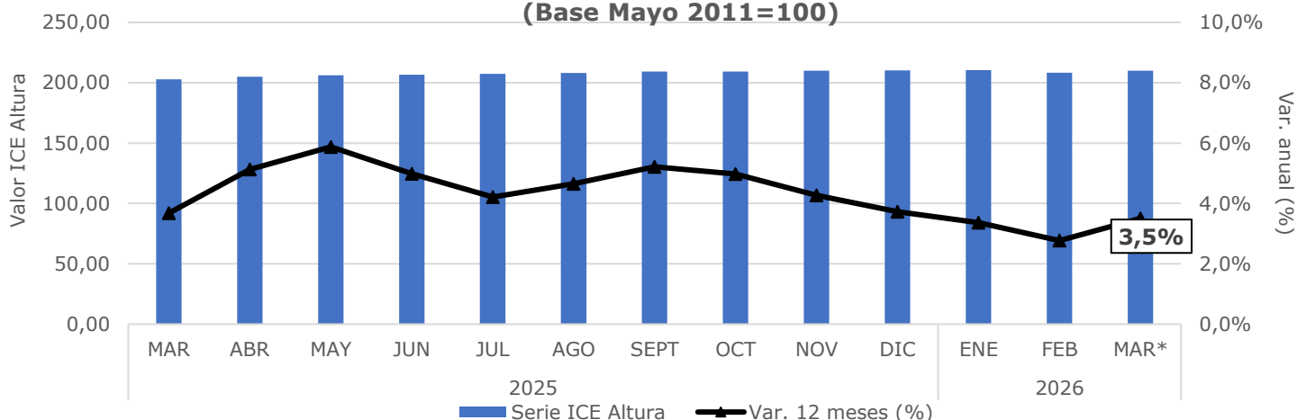
Índice Costo de Edificación en Altura Valor índice y variación porcentual respecto igual mes año anterior, período marzo 2025-marzo 2026 (Base Mayo 2011=100)
